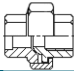
UNION 3P. F.GAZ x F.SW
