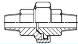
UNION 3P. M.GAZ x M.GAZ
