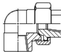
COUDE UNION F.GAZ x F.GAZ
