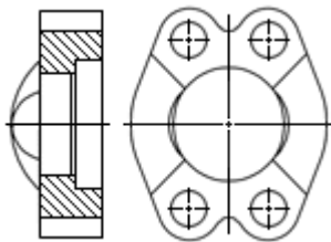
BRIDE MONOBLOC
