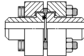
BRIDE LIAISON CETOP BWI
